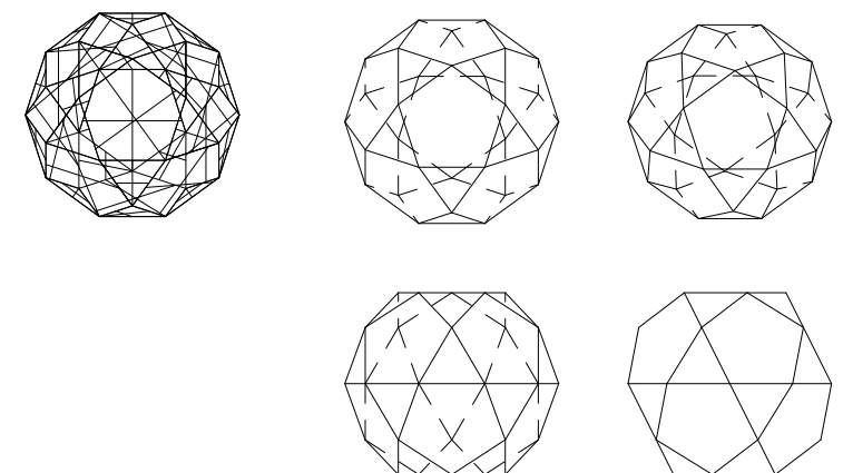
ICOSIDODECAEDRO
