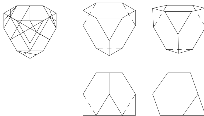
TETRAEDRO TRUNCADO
