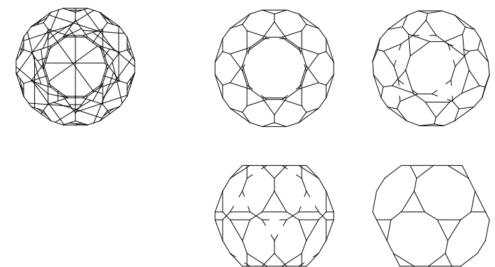
DODECAEDRO TRUNCADO
